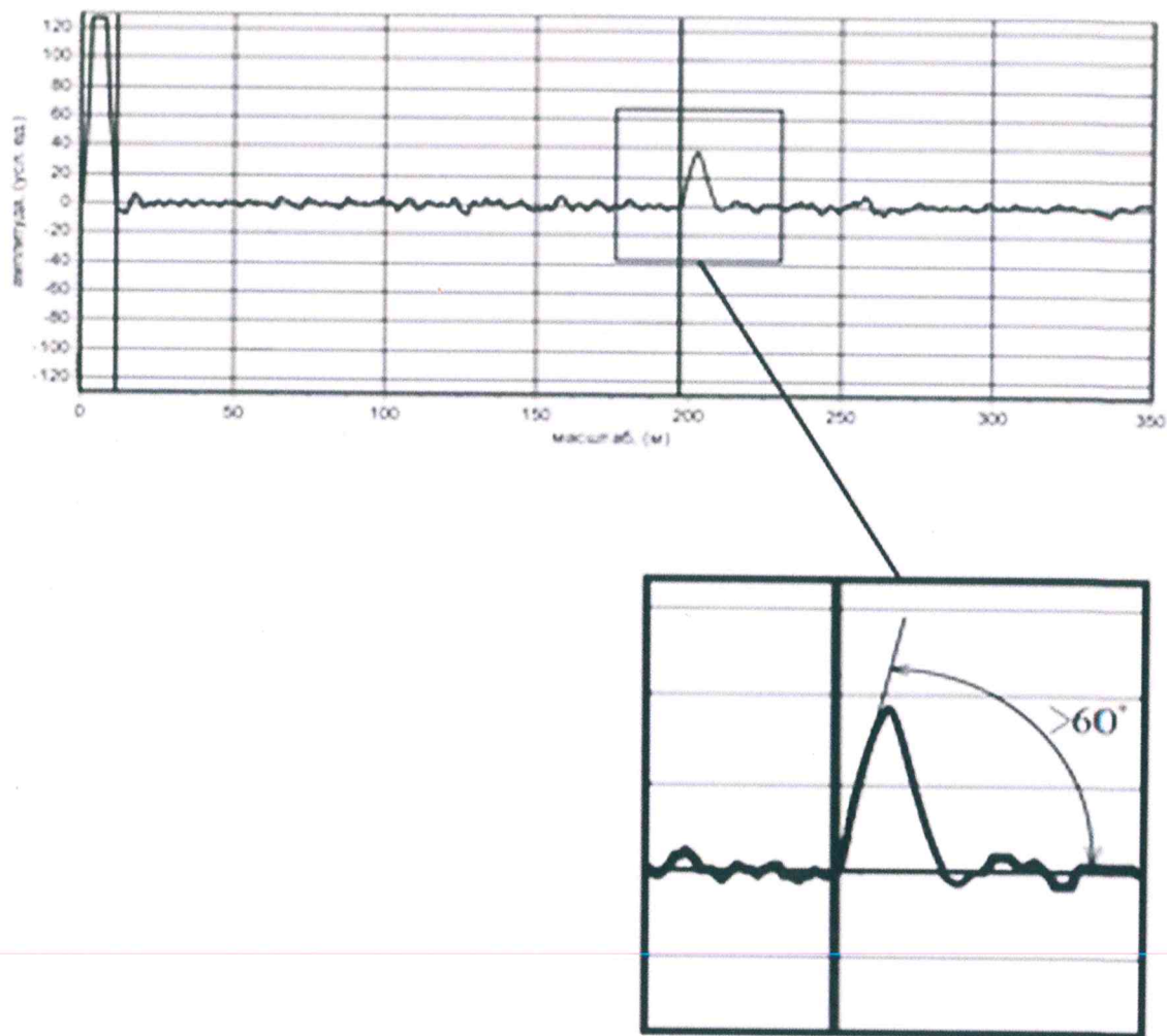
Рисунок 19. Параметры отраженного импульса на рефлектограмме.
