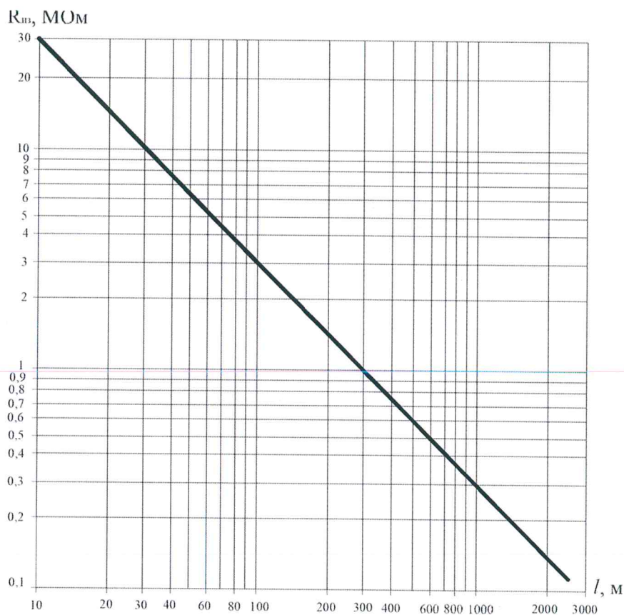
Рис. 1 Значение сопротивления изоляции в зависимости от длины сигнальной линии.
